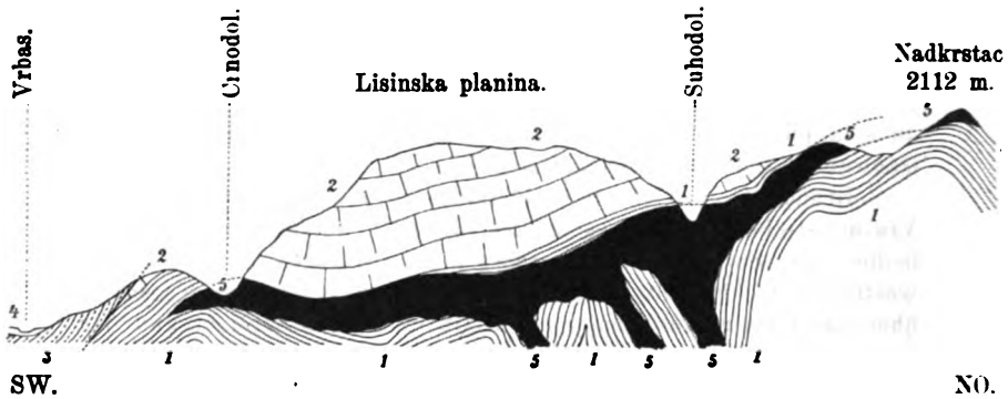
Fig. 2. Profil durch den Quarzporphyrerguß des Vratnica-Gebirges. 1 Karbonischer Phyllit. 2 Permokarbonischer Kalkstein. 3 Grödener (oberpermischer) Sandstein. 4 Diluvium und Alluvium. 5 Quarzporphyr. (Das Profil ist zweimal überhöht.)
